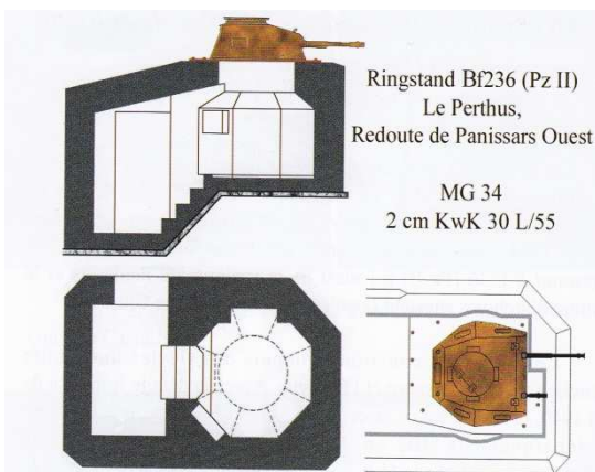
Cl. 5. Coupe et plans d'un Ringstand B-f 236 (Pz II) (DA Guillem Castellvi).
